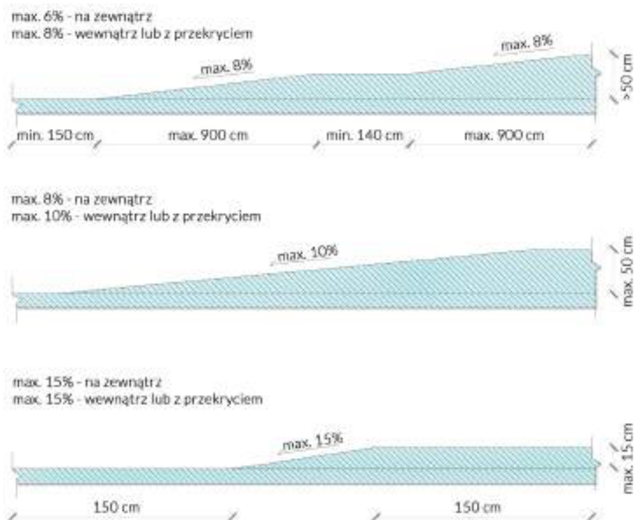
Rys. 39 Spadki pochylni zgodne z Warunkami Technicznymi
