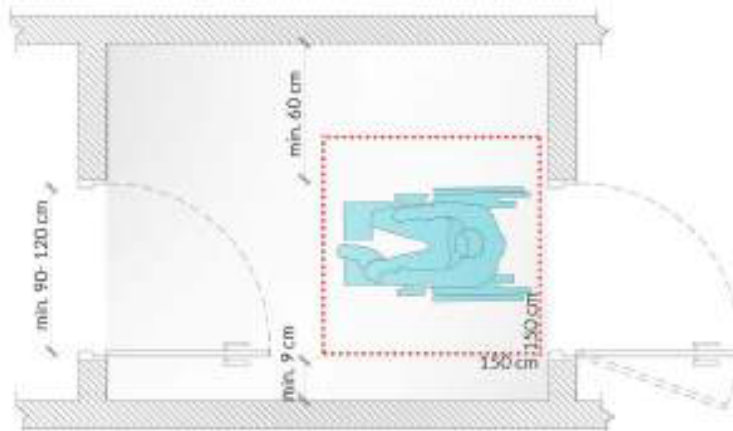
Rys. 15 Przykładowe rozwiązanie przestrzeni wiatrołapu z zapewnieniem niezbędnych wymiarów oraz przestrzeni manewrowej
