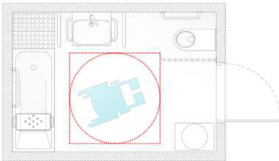
Rys. 52 Przykładowa aranżacja łazienki przystosowanej do potrzeb osób z niepełnościami
