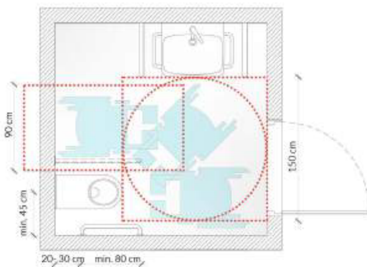
Rys. 54 Toaleta przeznaczona dla osób z niepełnosprawnościami
